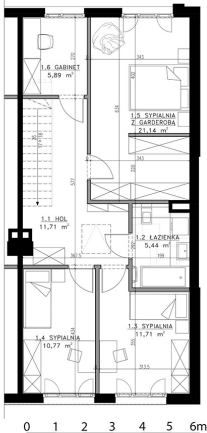
RZUT PIĘTRA
