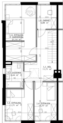
RZUT PIĘTRA
